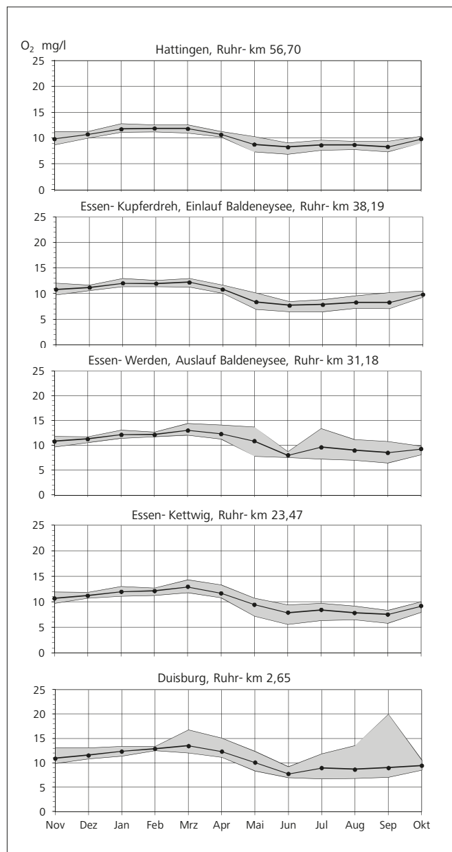
Bild 3.3: Sauerstoffgehalte in der Ruhr, monatliche Durchschnittswerte und Bandbreite der Tagesdurchschnittswerte, Abflussjahr 2016 Fig. 3.3: Oxygen in the Ruhr, monthly means and spread of daily means, water year 2016
