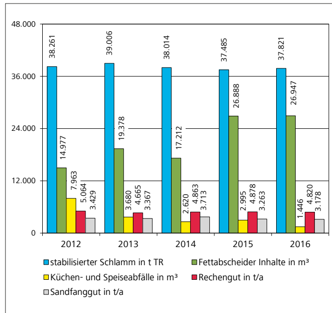
Bild 12.6: Reststoffmengen und angelieferte Co-Substrate der Jahre 2012 bis 2016 Fig. 12.6: Residue volumes and supplied co-substrates from 2012 to 2016
