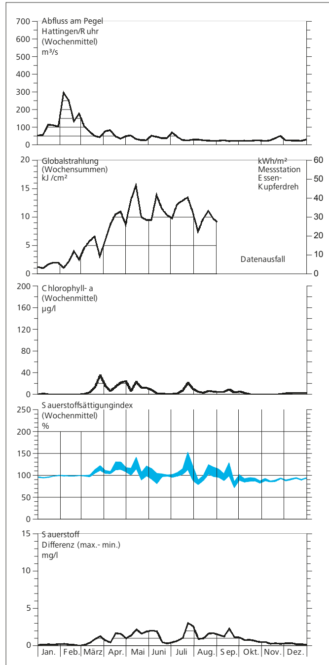
Bild 5.8: Einfluss der Wasserführung und der Globalstrahlung auf die Algenentwicklung im Baldeneysee und deren Auswirkung auf den Sauerstoffgehalt im Jahr 2016
