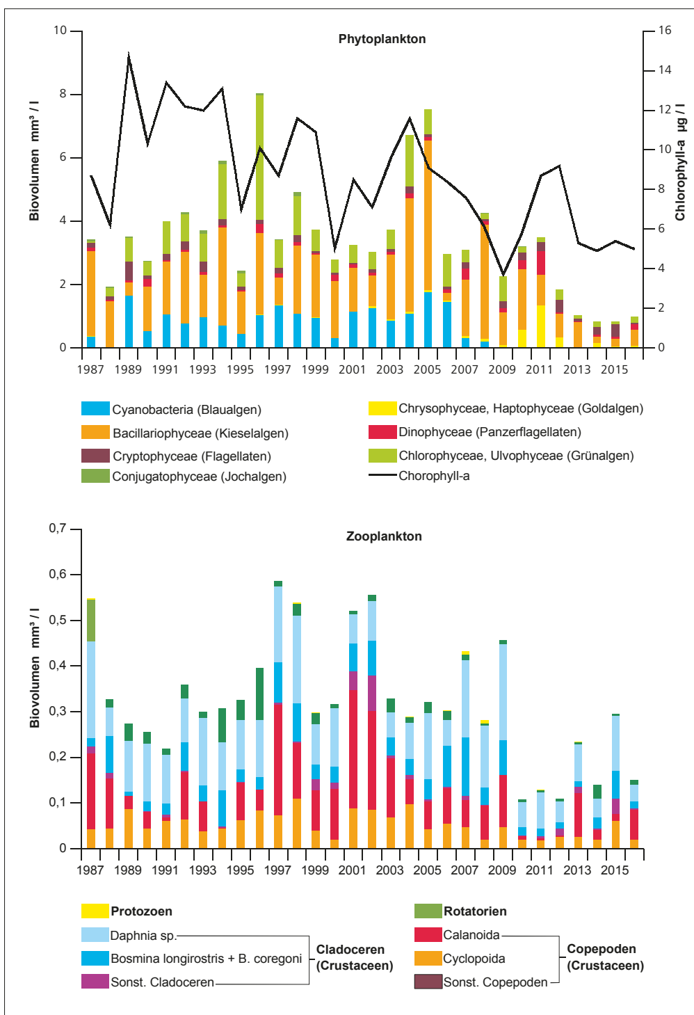
Bild 6.7: Phyto- und Zooplankton an der Probenahmestelle „Hen-netalsperre vor Damm“ in den letzten 30 Jahren (Jahresmittel)
