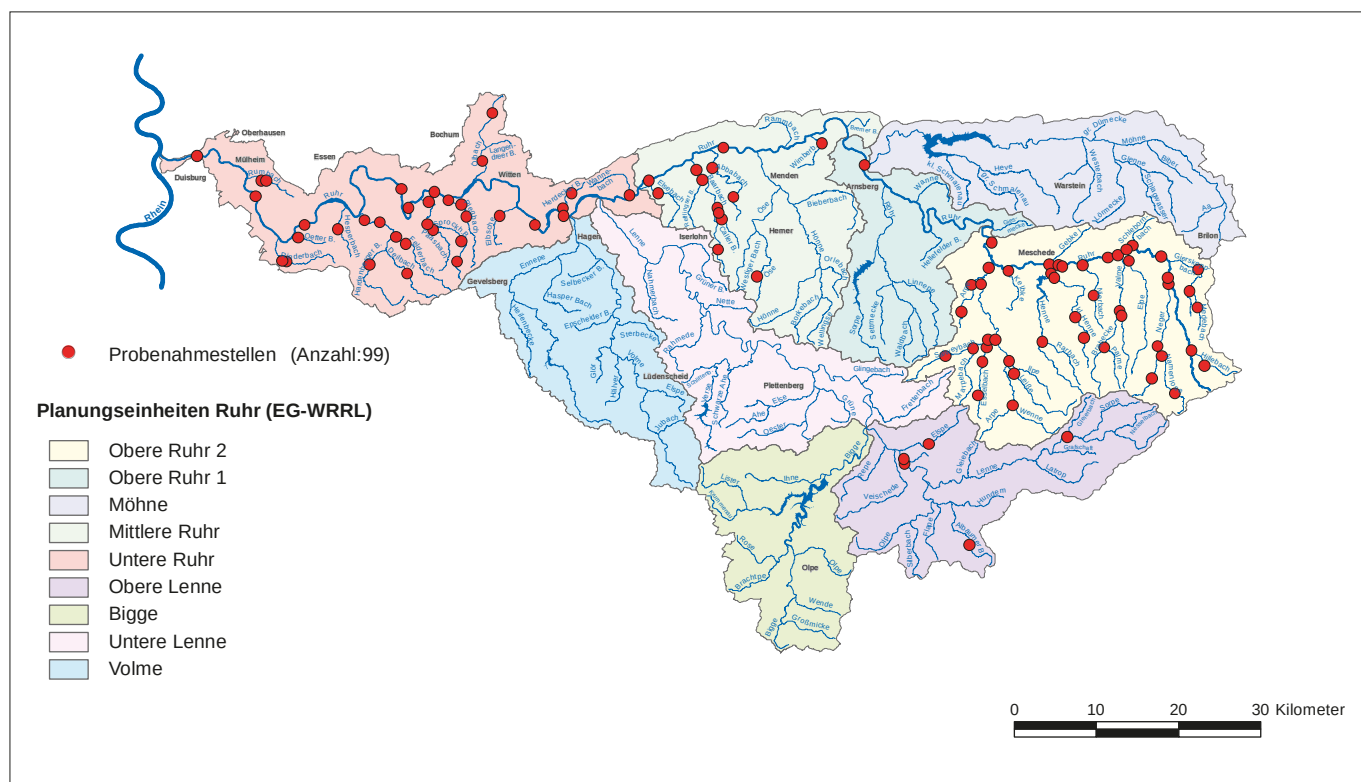
Bild 4.1: Lage der im Jahr 2015 und 2016 untersuchten Fließgewässer einschließlich der jeweiligen Probenahmestellen. Quelle: Geobasisdaten der Kommunen und des Landes NRW © Geobasis NRW 2015 Fig. 4.1: Location of the flowing waters monitored in 2015 and 2016 by Ruhrverband and LANUV including the respective sampling points. Source: Geobasisdaten der Kommunen und des Landes NRW © Geobasis NRW 2015
