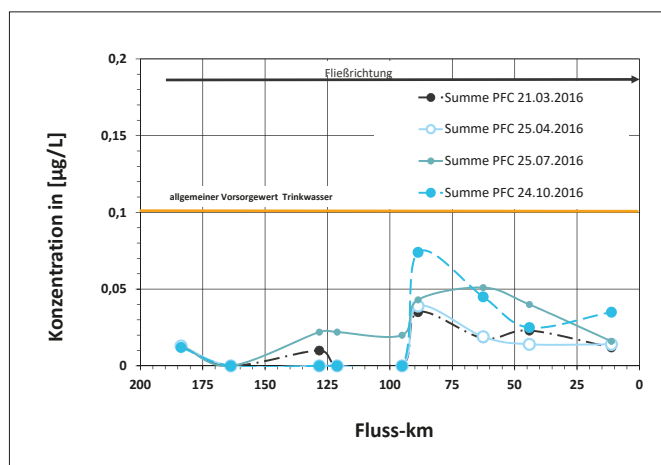
Bild 15.2: Summierte Konzentrationen per- und polyfluorierter Verbindungen in Untersuchungen des Oberflächenwassers im Jahr 2016 im Ruhrflängsverlauf
