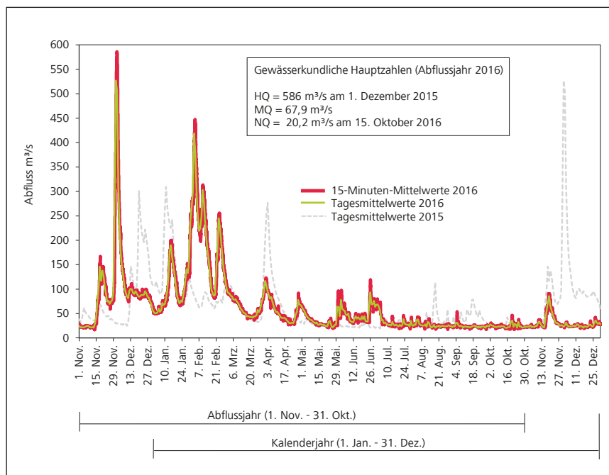
15-Minuten-Mittelwerte und Tagesmittelwerte des Abflusses der Ruhr am Pegel Hattingen/ Ruhr im Abfluss- und Kalenderjahr 2016 Runoff means during 15 minutes and 24 hours at the gauging station Hattingen/Ruhr in the water year and calendar year 2016
