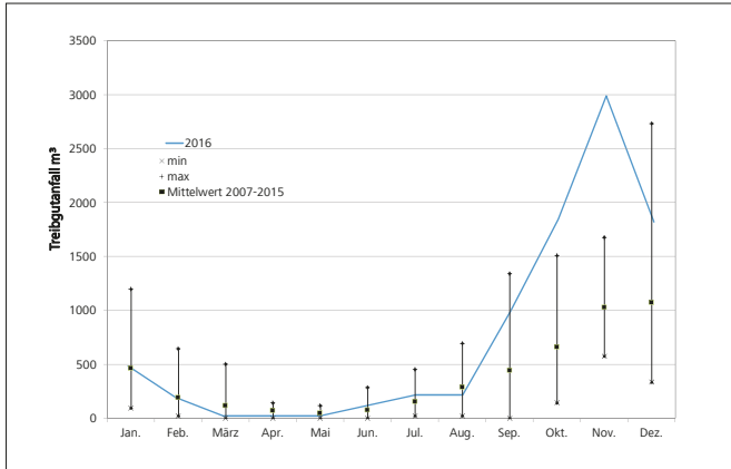
Bild 5.19: Mittelwerte des monatlichen Treibgut anfalls [m³] mit Minimum- und Maximum-Werten an der Rechenanlage des Wasserkraftwerks am Hengsteysee im Zeitraum 2007 bis 2015 sowie der zeitliche Verlauf der Treibgutmengen für das Jahr 2016
