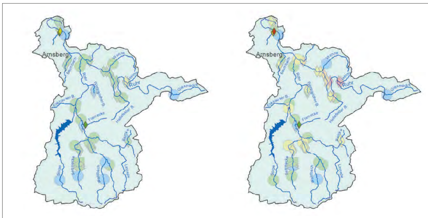
Bild 4.6: Ökologischer Gewässerzustand – Makrozoobenthos, Ausschnittskarten der Planungseinheit Obere Ruhr 1 (PE 1600). Links: Modul Saprobie, rechts: Modul Allgemeine Degradation. Kleine, intensiv gefärbte Symbole = 2016, große, schwach gefärbte Symbole = 2011 bis 2015. Quelle (Karte): Land NRW (2017) Datenlizenz Deutschland – Namensnennung – Version 2.0 ( www.govdata.de/dl-de/by-2-0 )
