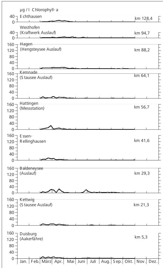
Bild 5.7: Algenentwicklung (als Chlorophyll-a-Gehalt) an verschiedenen Stellen der Ruhr im Verlauf des Jahres 2016
