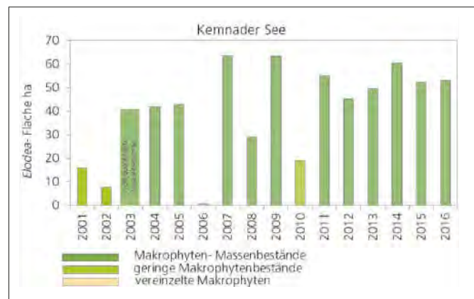
Bild 5.11: Bestandsflächen von Elodea nuttallii im Kemnader See in den Jahren 2001 bis 2015 (Daten auf Basis von Satelliten- und Luftbildauswertungen sowie Vor-Ort-Kartierung, 2008, 2012, 2014, 2015 und 2016 Bestände durch Mahd reduziert)
