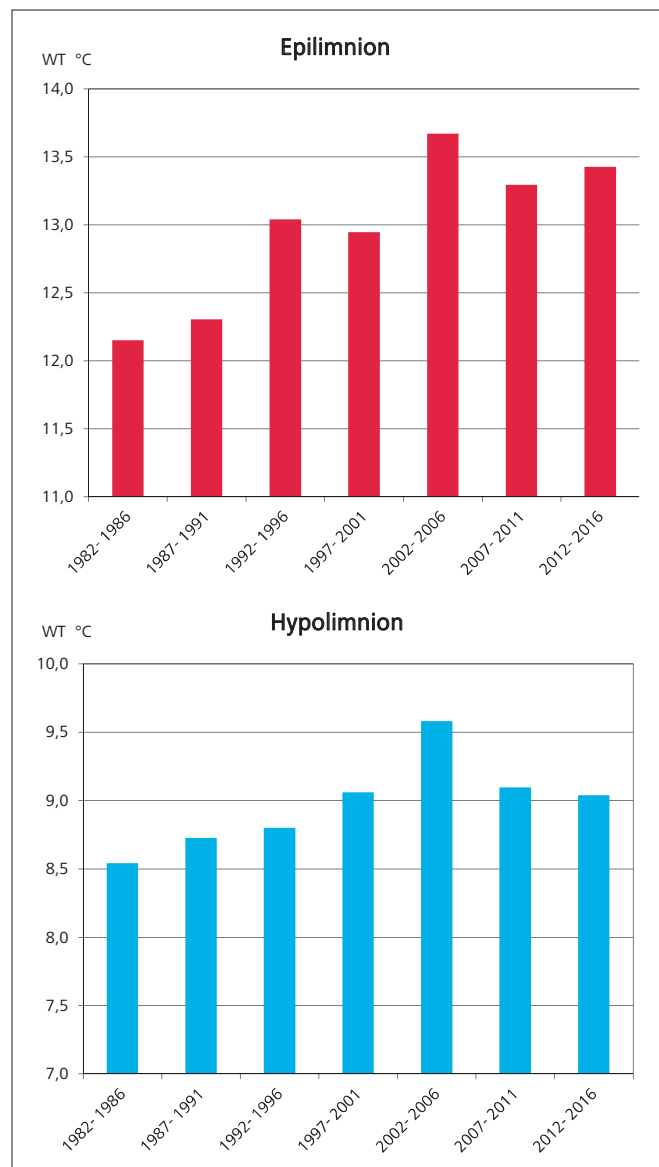
Bild 6.2: Mittlere epi- und hypolimnische Wassertemperaturen in der Möhnetalsperre in den letzten 35 Jahren Fig. 6.2: Mean epilimnetic and hypolimnetic water temperatures in the Möhne Reservoir during the past 35 years
