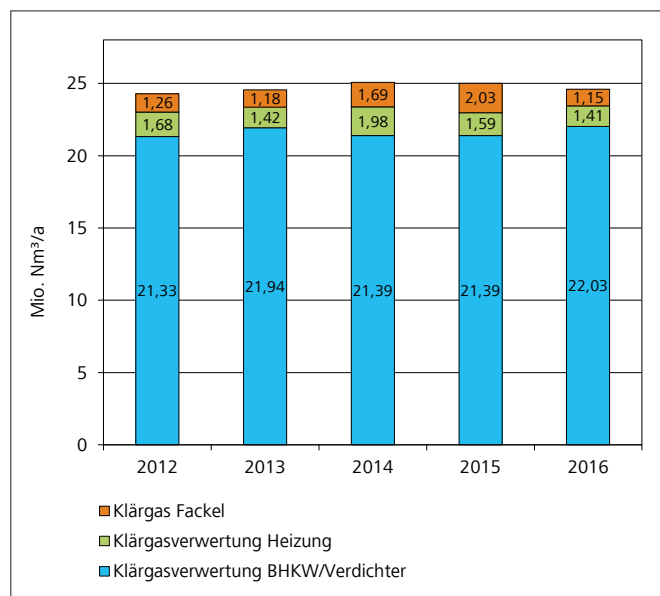
Bild 12.7: Klärgasverwertung auf den Ruhrverbandskläranlagen von 2012 bis 2016 Fig. 12.7: Sewage gas utilisation at the Ruhrverband's sewage treatment plants from 2012 to 2016
